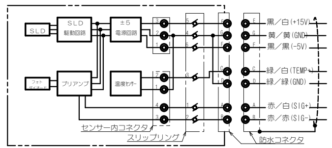
接続図
